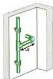
ج : با ایجاد یک خم L شکل در قسمت انشعاب رایزر اجازه حرکت محوری به رایزر داده شود
